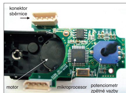
Obr. 3. Pohled na vnitřní uspořádání pohonu ze strany odvrácené od hřídele s vyklopenou deskou plošného spoje
