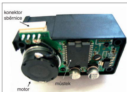
Obr. 2. Pohled na pohon ze strany odvrácené od hřídele
