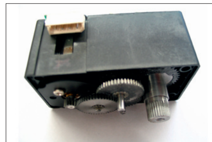
Obr. 4. Pohled na pohon bez krytu ze strany hřídele
