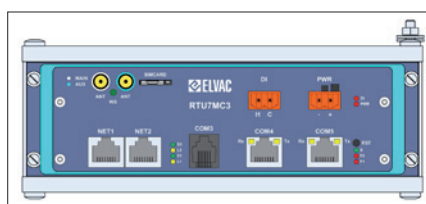
Obr. 3. Komunikační jednotka (router) RTU7MC3
