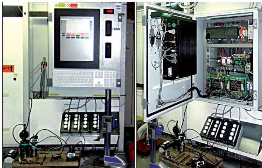
Obr. 3. Pracoviště mezioperační kontroly kvality v Aerocan CZ
